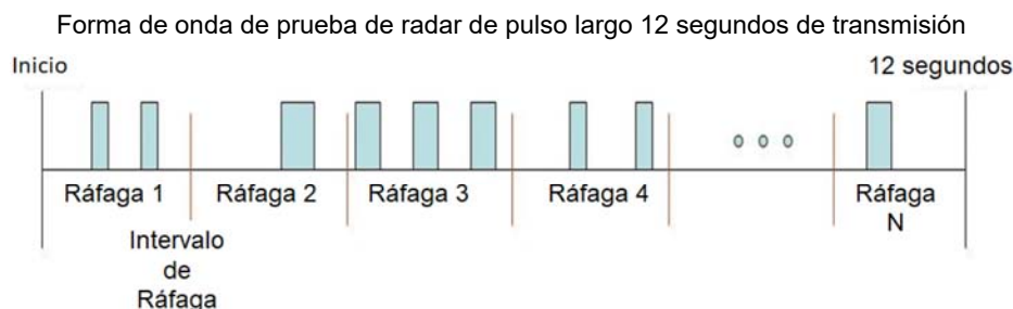
Figura 3. Representación gráfica de una forma de onda de tipo radar de Pulso largo
