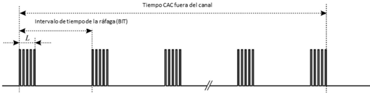
Figura 2E: Estructura general de la señal de prueba de radar de múltiples ráfagas/ basada en paquetes con PRF escalonado.
