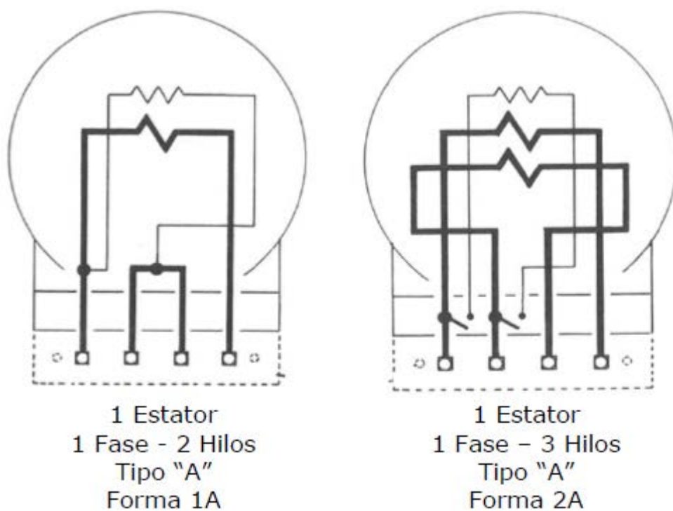
Figura 3 - Conexiones internas para wathorímetros tipo "A" monofásicos (vistas frontales)
