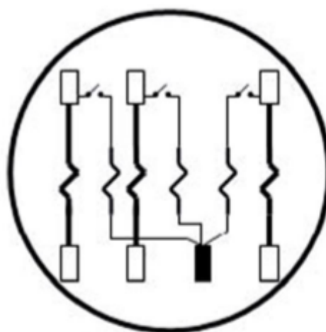
3 Estatores 4 Hilos y Estrella Forma 16 S
