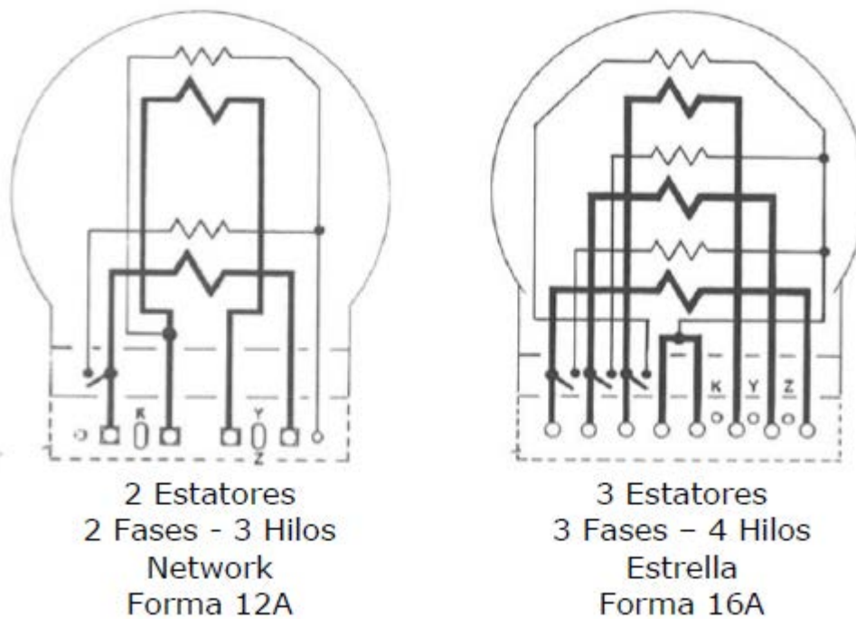
Figura 4 - Conexiones internas para wathorímetros, autocontenidos tipo "A" de varios estatores (vistas frontales)
