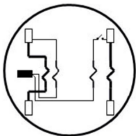
2 Estatores 3 Hilos Forma 12 S
