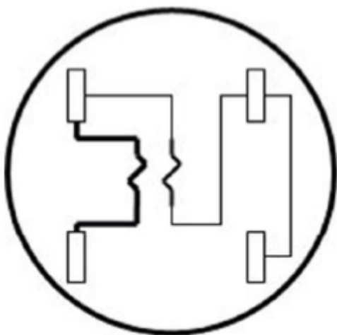
2 Hilos Auto contenido Forma 1 S
