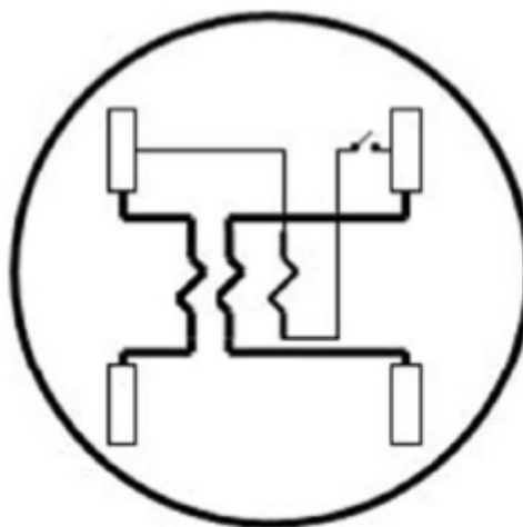
3 Hilos Auto contenido Forma 2 S
