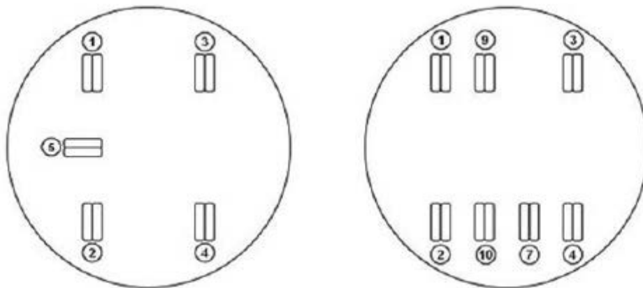
Figura 5 - Identificación de la posición de las mordazas de sujeción del wathorímetro una base enchufe
