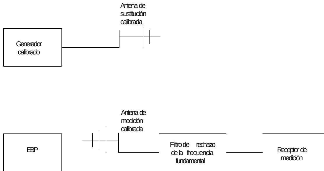
Figura 5.- Configuración para la medición de la p.i.r.e. de emisiones no esenciales
