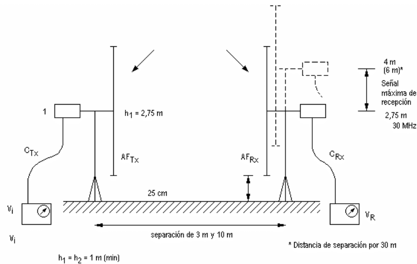
Figura A.2.- Sitio de prueba al aire libre con dos antenas orientadas vertical y horizontalmente con respecto a tierra
