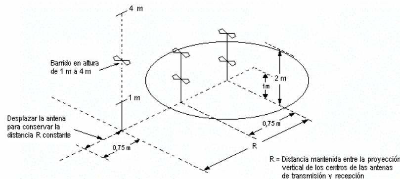
Figura A.6.- Validación del sitio al aire libre
