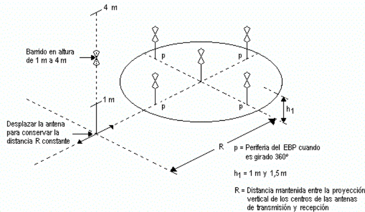
Figura A.3.- Polarización horizontal y vertical
