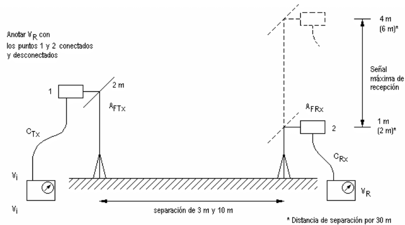
Figura A.1.- Sitio de prueba al aire libre con dos antenas orientadas vertical y horizontalmente con respecto a tierra
