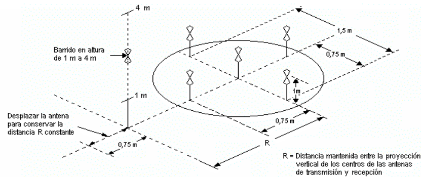
Figura A.5.- Validación del sitio al aire libre
