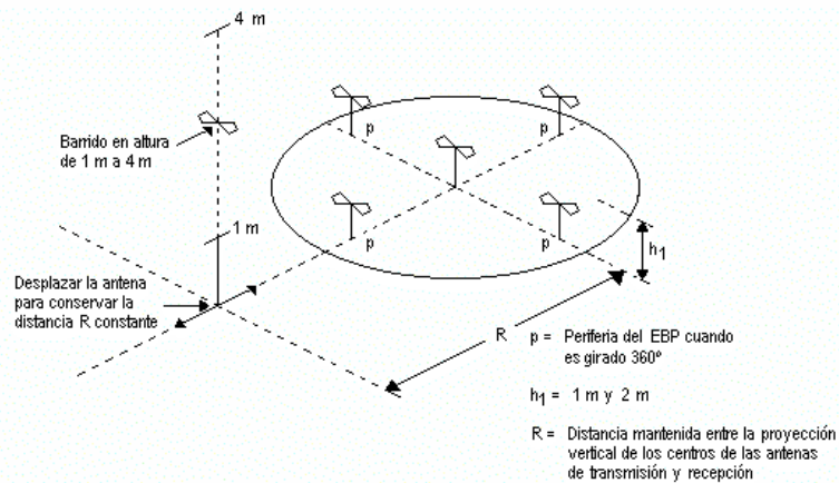
Figura A.4.- Polarización horizontal y vertical
